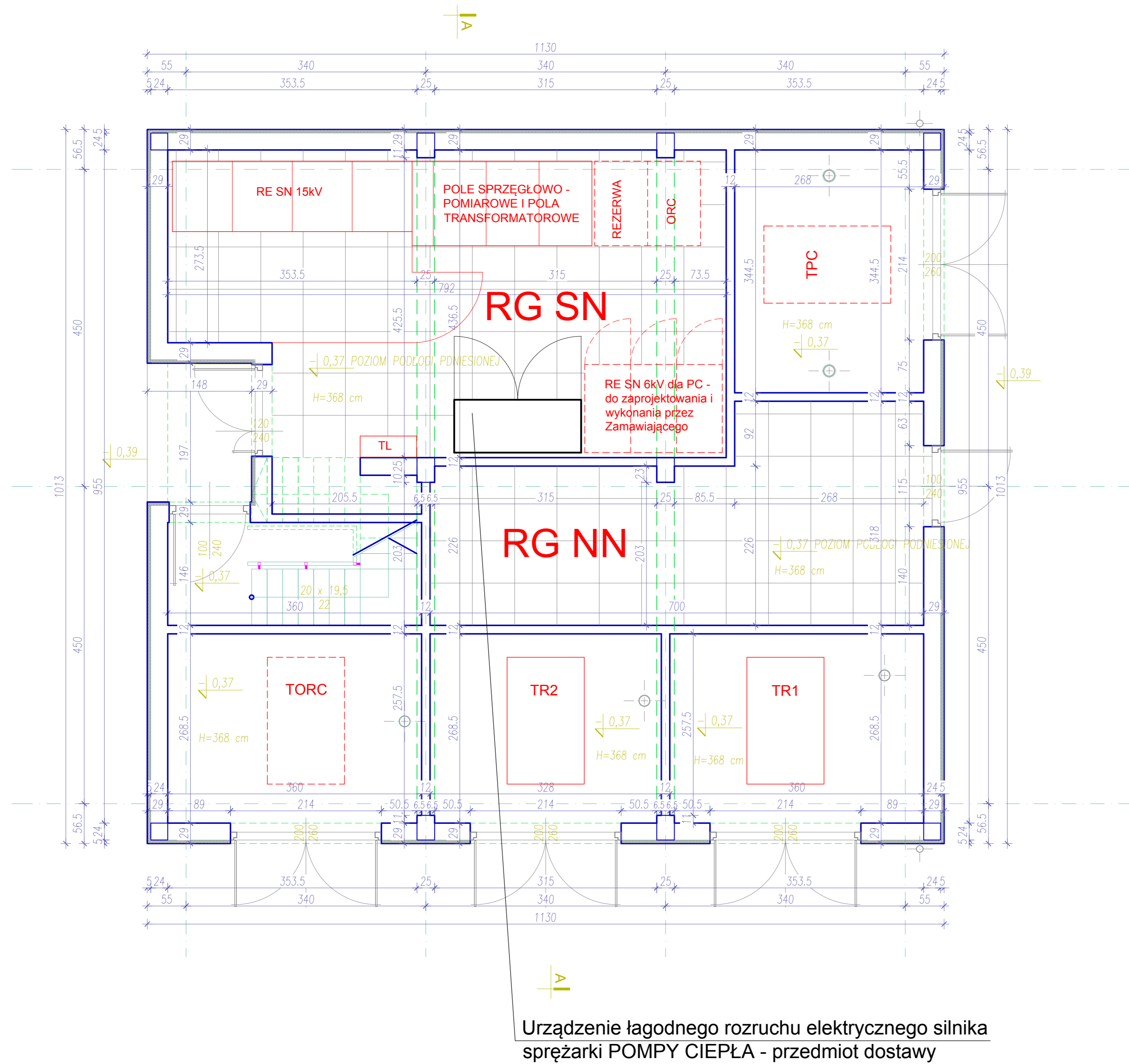
Rzut parteru
